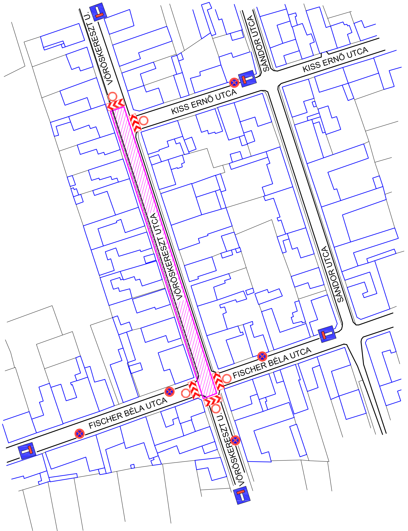
TERVEZETT FORGALOMKORLÁTOZÁS KEHOP-2.1.11 - VÍZIKÖZMŰ HÁLÓZATOK ÁTALAKÍTÁSA ÉS HATÉKONYSÁGNÖVELŐ FEJLESZTÉSE PÉCSETT 1. RÉSZ - VÖRÖSKERESZT UTCA VÍZ ÉS SZENNYVÍZ REKONSTRUKCIÓ I. ÜTEM - TELJES ÚTZÁR - 2023.08.21. - 2023.09.29.
